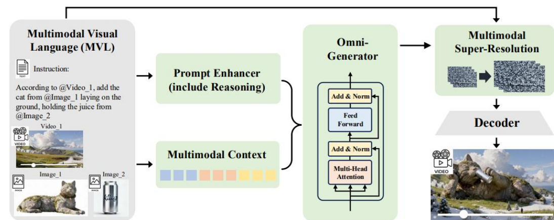
图: Kling-Omni架构
