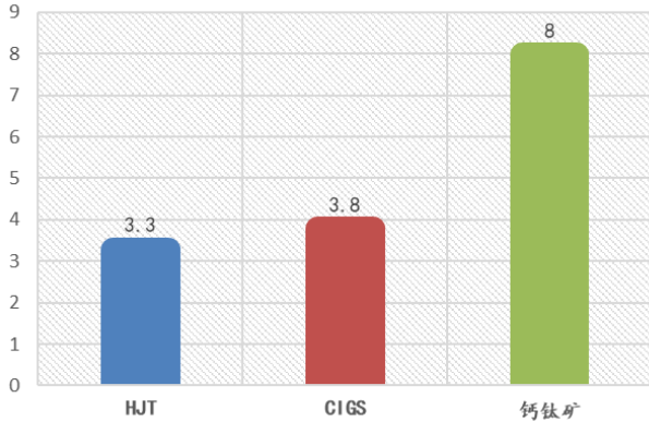
图48: 各类太阳能电池单位耗钢量 (吨/GW)
