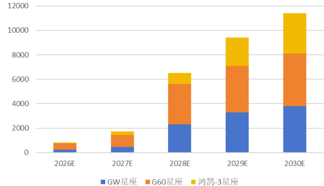
图19: 2026-2030 年间中国三大低轨卫星互联网星座发射量预测 (颗)
